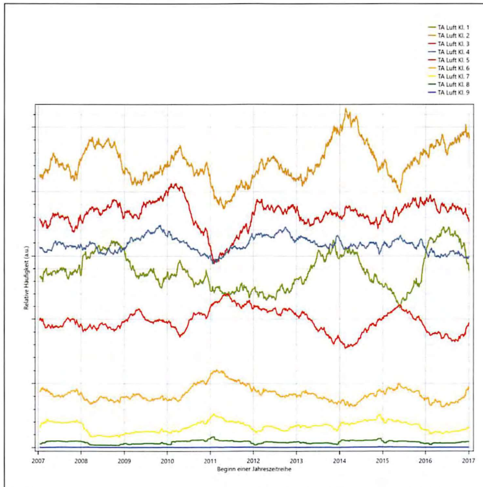
Abbildung 18: Prüfung auf vollständige und homogene Daten der Windmesstation anhand der Windschwindigkeitsverteilung
